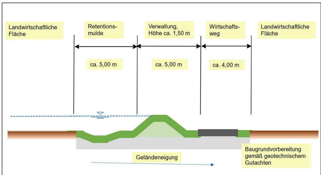
Abb. 6-2: Ortsgemeinde Minfeld, Schema der Dammanlage im Querprofil
