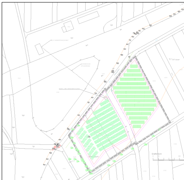
Abbildung 1 Geltungsbereich mit Modulen (Vorentwurf)
