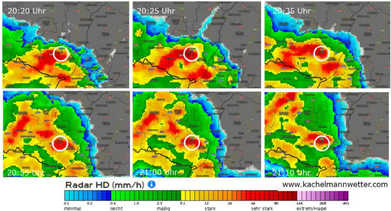
Abb. 4-1: Regenradarauswertung Starkregenereignis vom 28.07.2014 [13]
